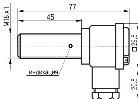
Габаритный чертеж.
